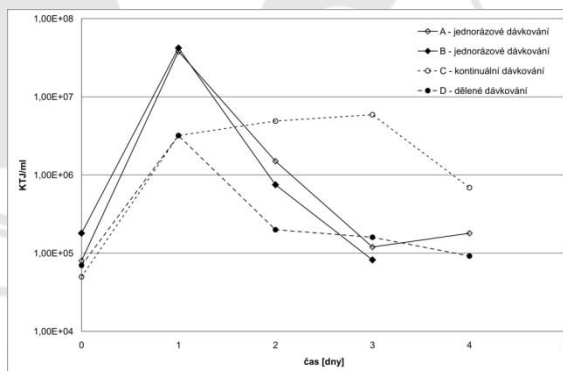
Obr. č. 2 Průběh koncentrace HMO v inokulu při testu způsobu dávkování nutričních a C-zdroje
