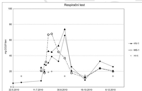
Obr. č. 5 Průběh respirační aktivity MO v p.v. (laboratorní respirační test)
